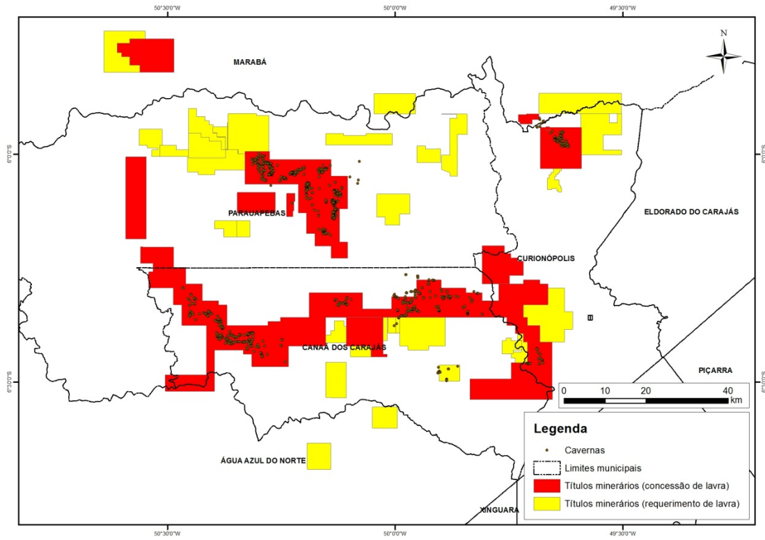
Figura 3. Cavernas e títulos minerários na região de Carajás (elaborado pelo autor)
