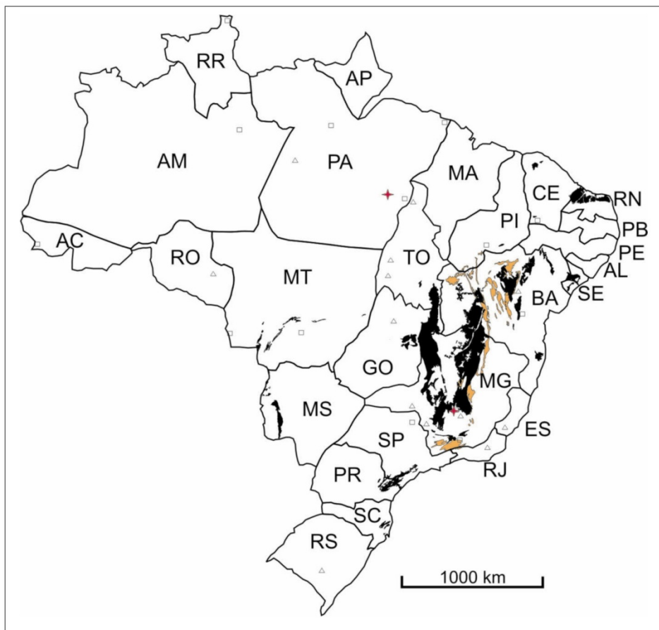
Figura 1. Mapa com as principais litologias que apresentam cavernas. Rochas carbonáticas estão representadas em preto. Rochas siliciclásticas estão representadas em laranja. As principais áreas de canga e formação ferrífera que apresentam cavernas estão representadas por estrelas vermelhas. (Piló & Auler, 2013)
