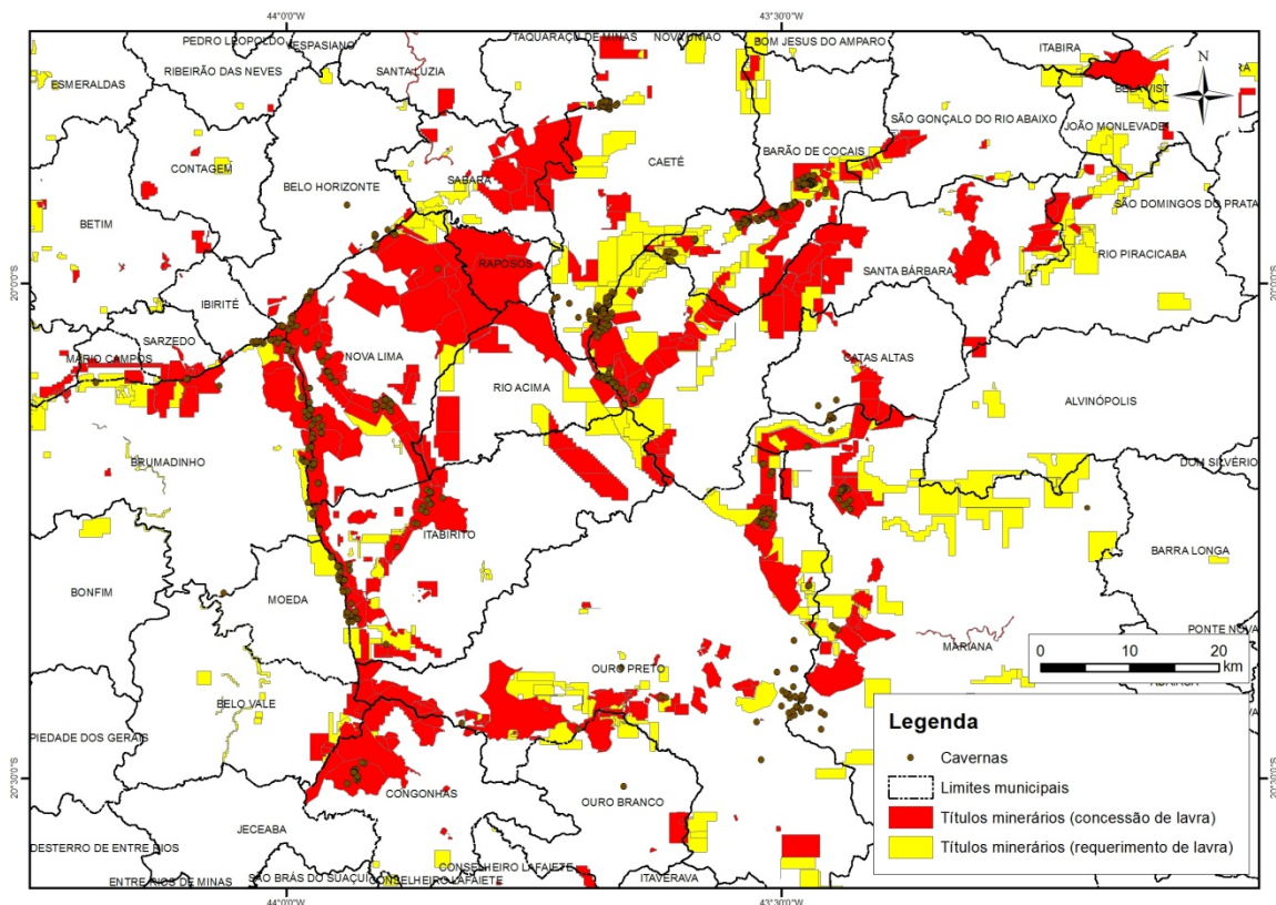
Figura 5. Cavernas e títulos minerários na região do Quadrilátero Ferrífero (elaborado pelo autor)
