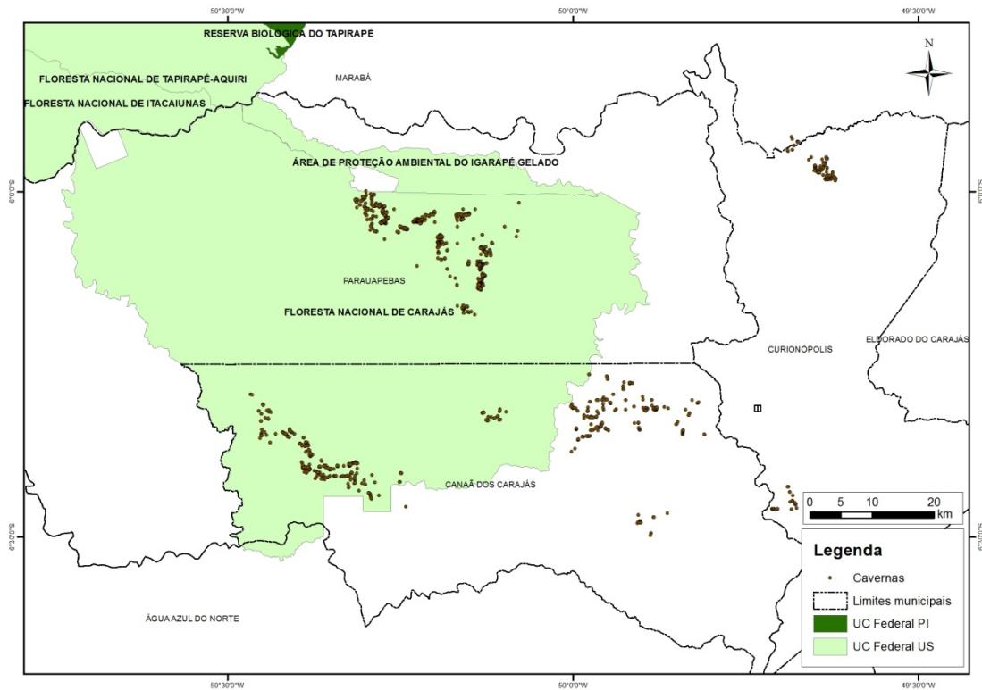
Figura 4. Cavernas e unidades de conservação na região de Carajás (elaborado pelo autor)
