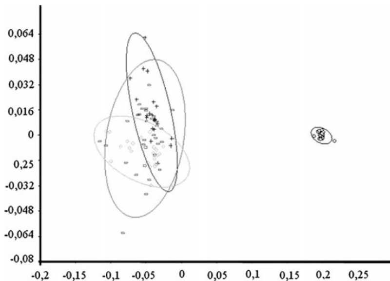
Figura 2. Gráfico de escalonamento multidimensional não métrico (MDS) mostrando a composição de espécies em cavernas abrigadas em rochas carbonáticas (+), siliciclásticas (◇), ígneas (□) e ferríferas (○). (Silva et al., 2011).
