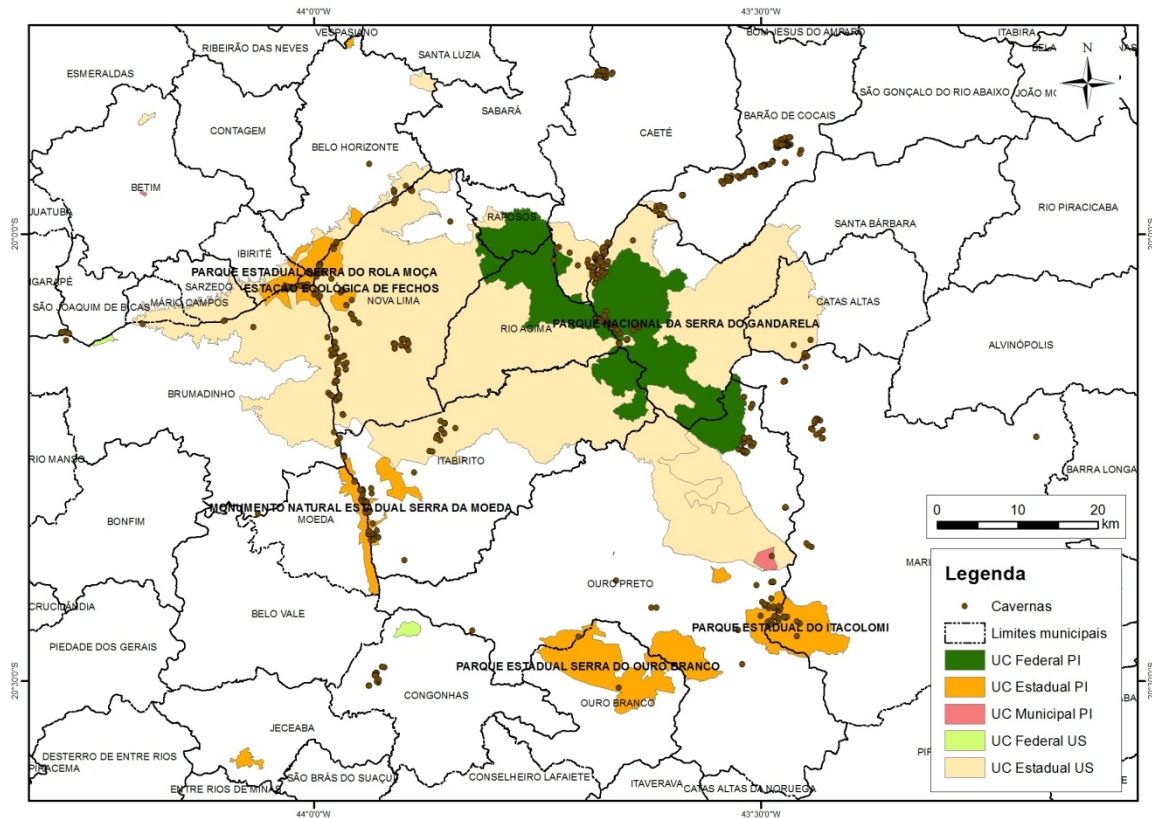
Figura 6. Cavernas e unidades de conservação na região do Quadrilátero Ferrífero (elaborado pelo autor)
